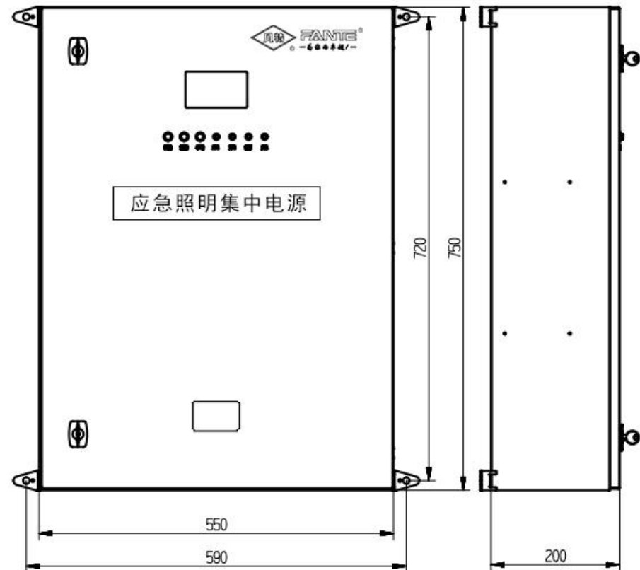
图1 应急照明集中电源外形示意图
